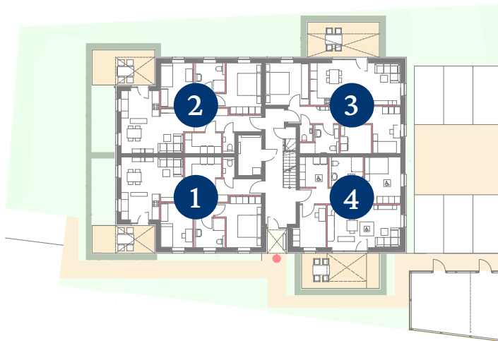
Erdgeschoss
